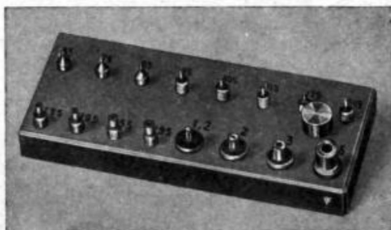
Die Anbögen und Preßstempel zum Apparat
