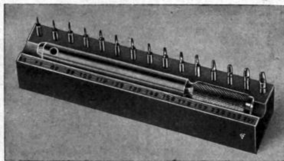
Die Spezial-Reibglättfahlen zum Apparat
