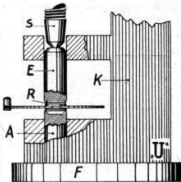
Der Querschnitt des praktischen Apparates
