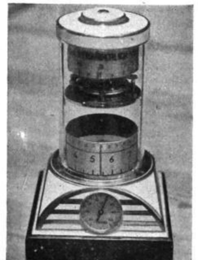
Instrument zum Messen von Zeit, Luftdruck und Temperatur
