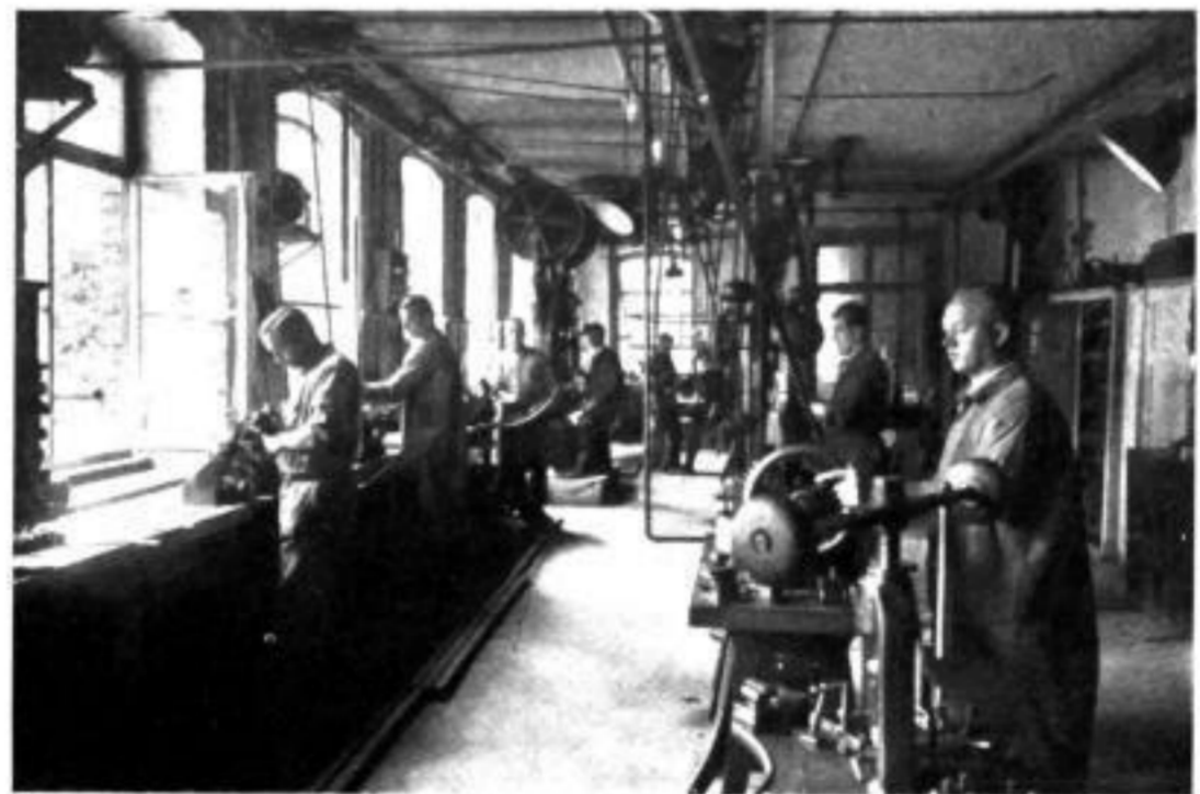
Die Einzelteile der Uhrengehäuse werden vorgearbeitet
