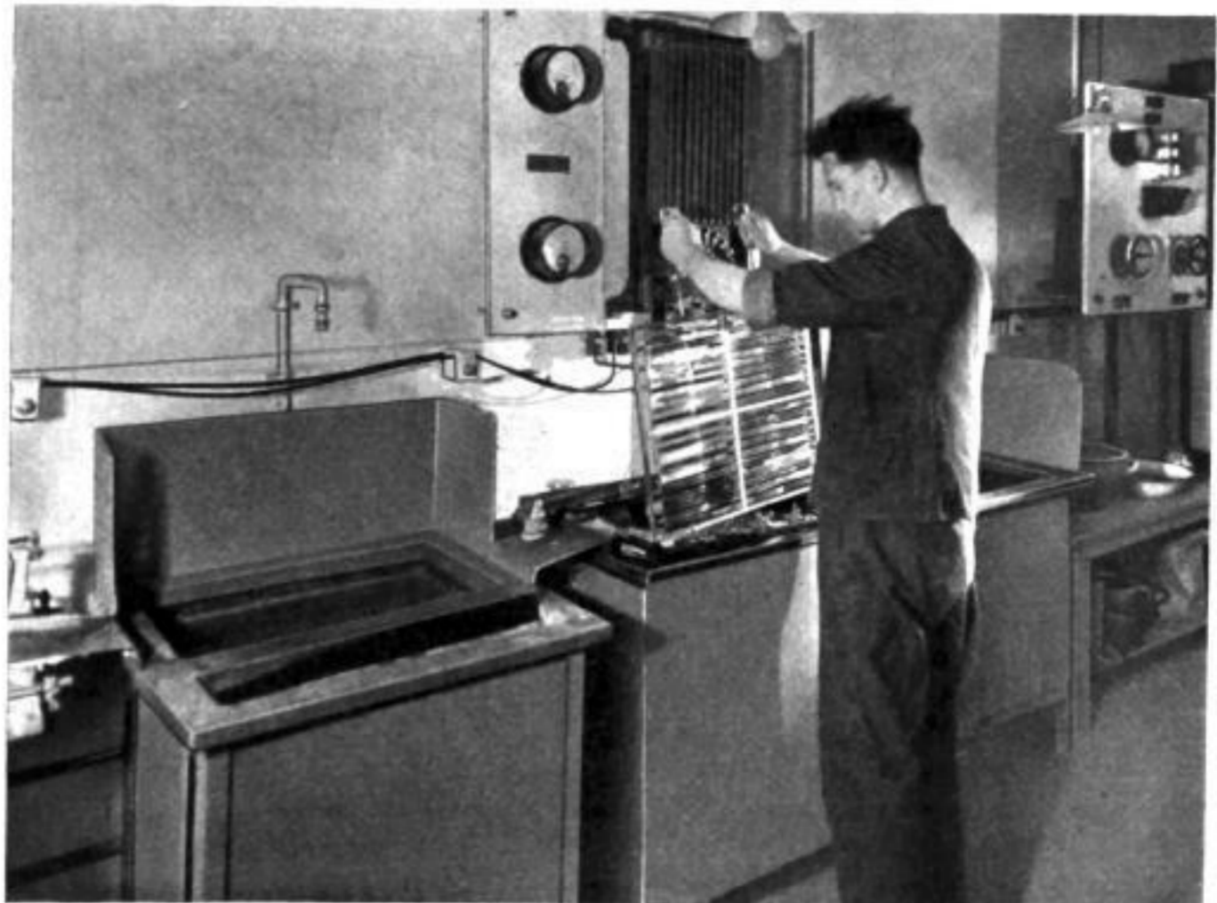
Teilbild der Verchromungsanlage. Die Metall-Uhrarmbänder werden vor der Verchromung erst vernickelt, um die Haltbarkeit und Dauerhaftigkeit der Bänder zu erhöhen.
