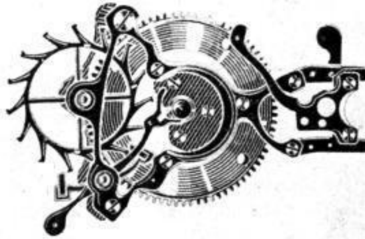
Teile der Drehganguhr mit Ankerhemmung. (Im Besitz des Führers.)
