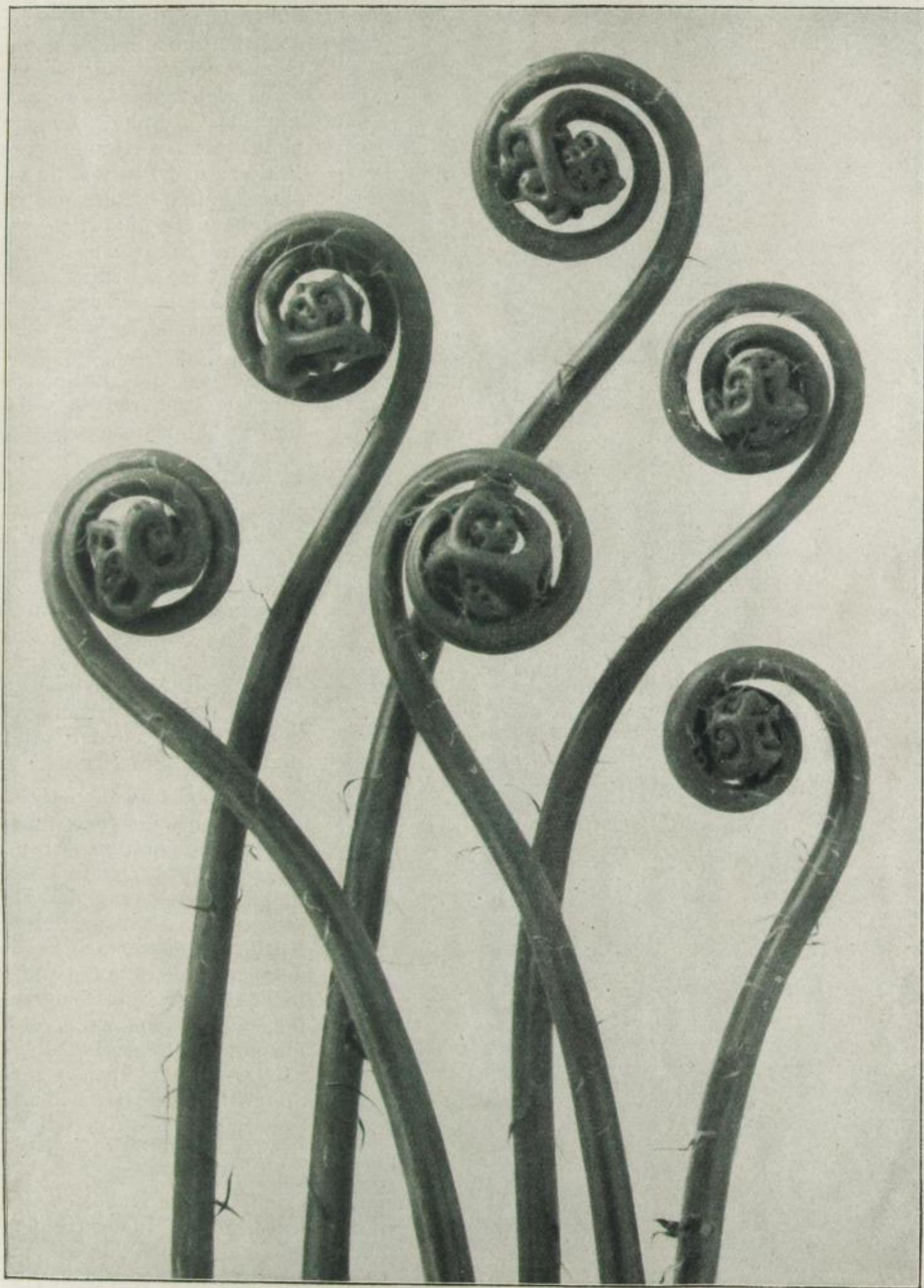
Die „Bischofstäbe“, mit denen das junge Blattgefieder des Farns alljährlich die Erde durchbricht (fünffache Vergrößerung).
