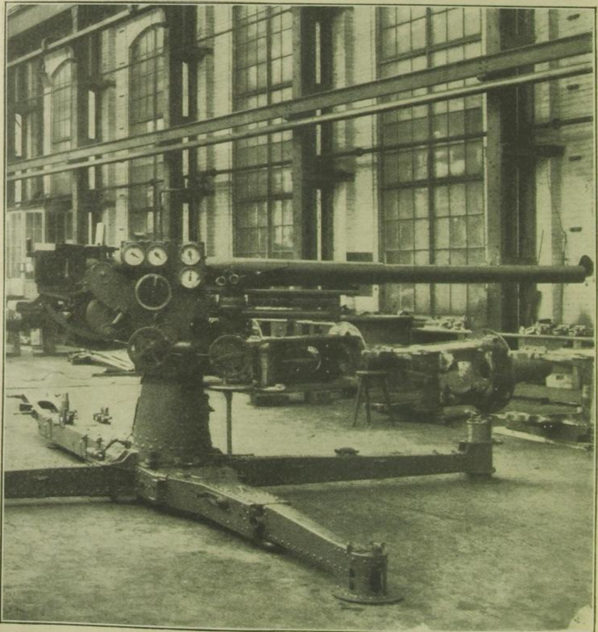
8-cm-Luftabwehrkanone, die den chemischen Vergiftungskrieg unwirksam machen soll.
