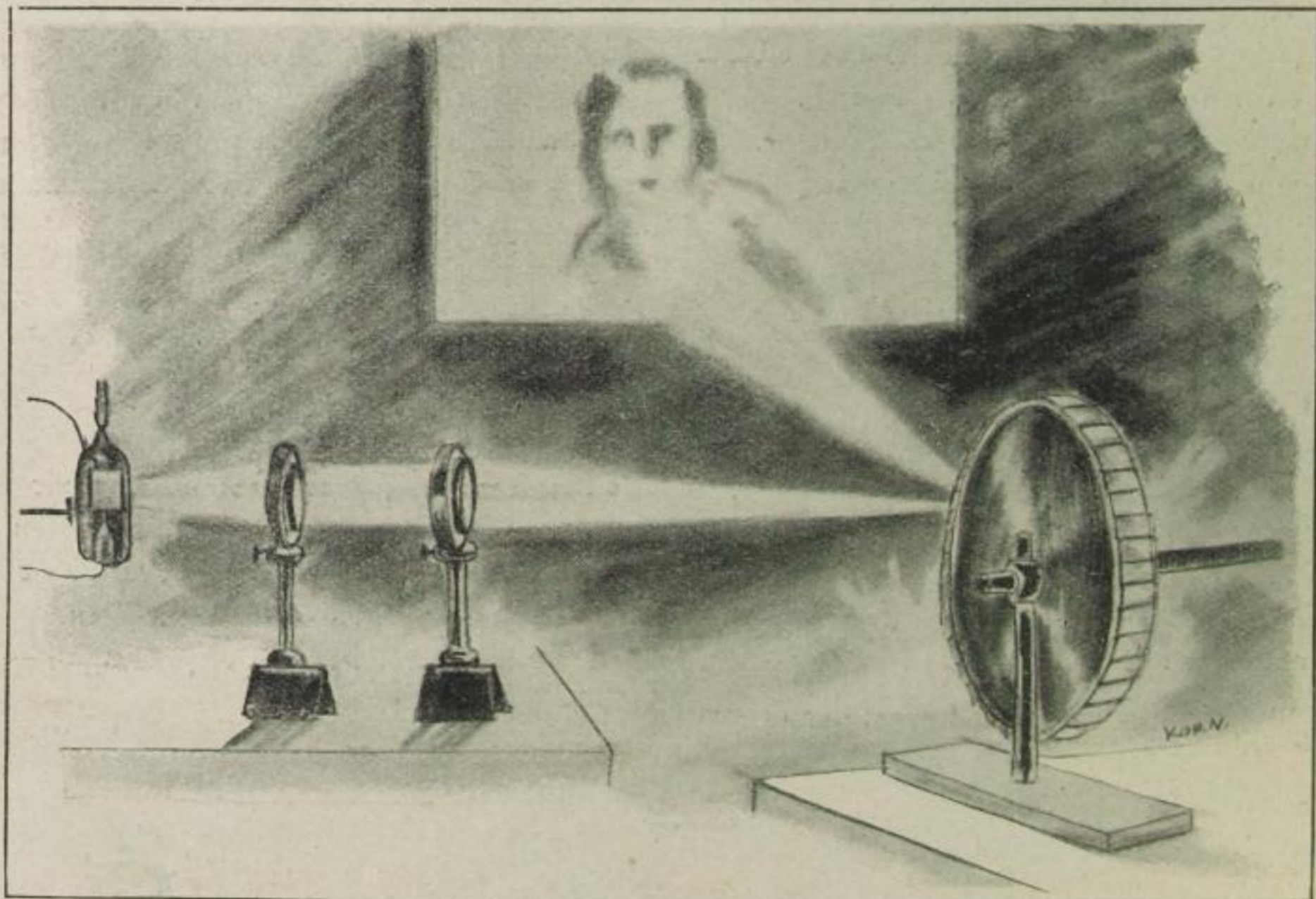
Fernseh-Empfang mit Weillerschem Spiegelrad
