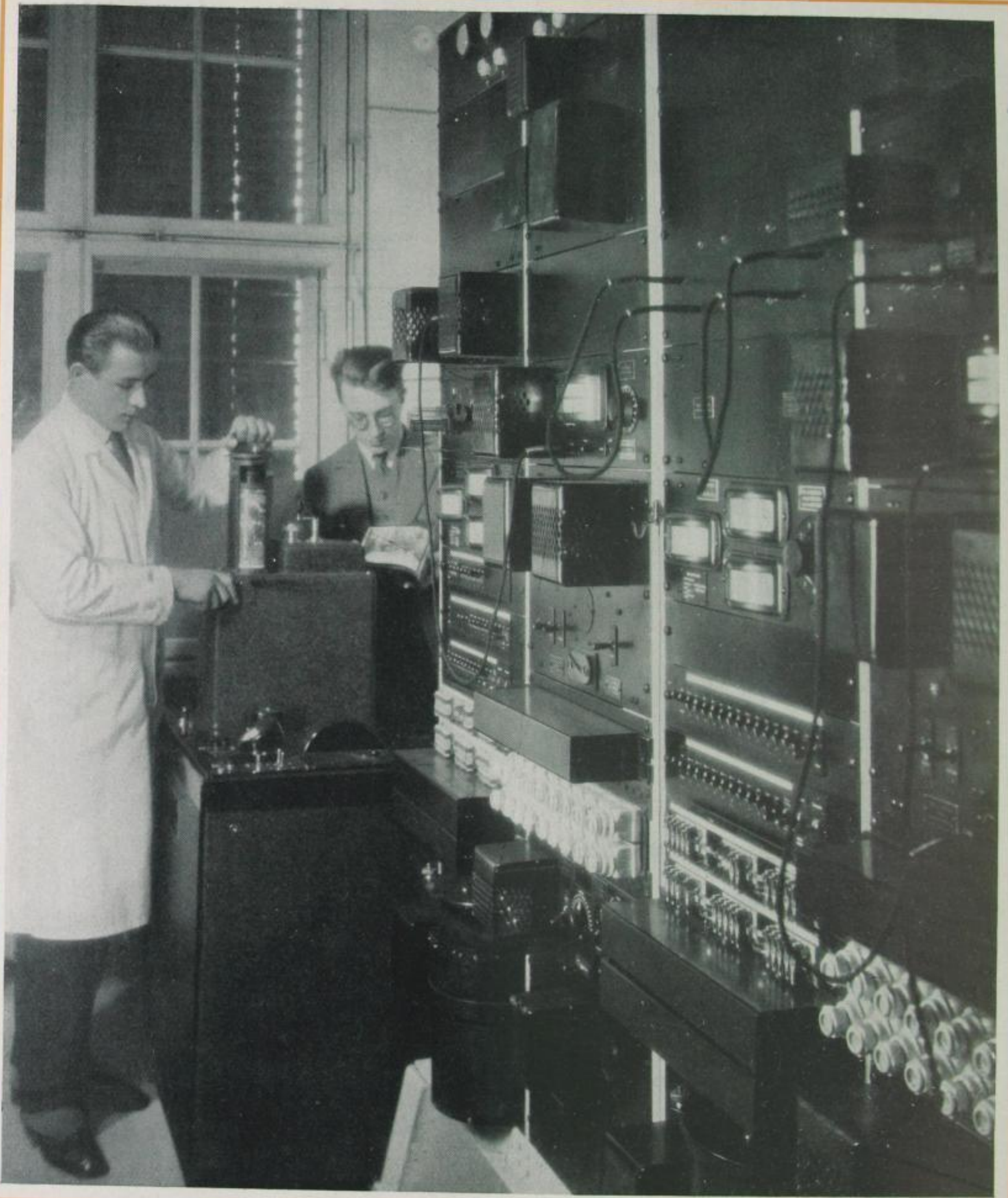
BILDTELEGRAFIE-STATION DES VERLAGES ULLSTEIN SYSTEM SIEMENS-KAROLUS-TELEFUNKEN
