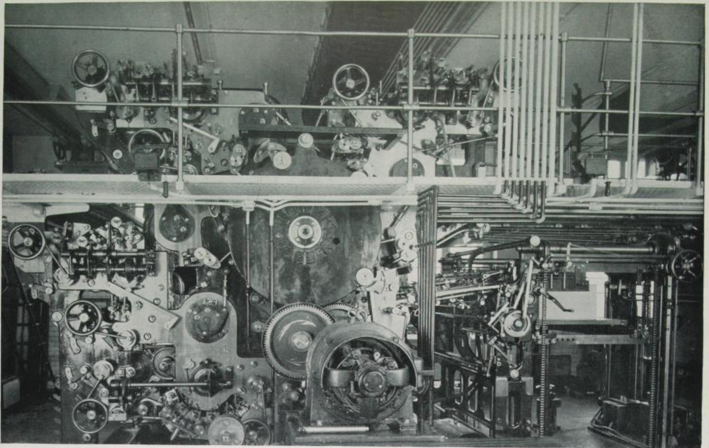
Eine Offset-Spezialmaschine, die im sogenannten „Naß-auf-Naß-Druckverfahren“ Papierbogen in einem Arbeitsgang vierfarbig bedruckt.
