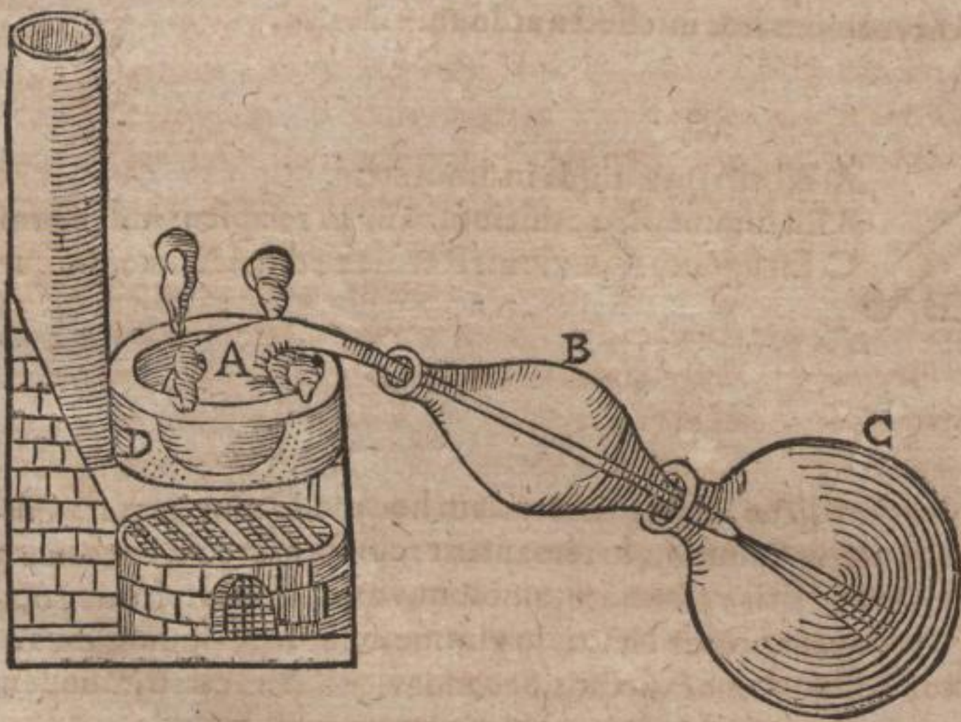
A. Retorta. B. Vesica. C. Recipiens. D. Vas terreum cineribus impletum, in quod Retorta A. adaptatur.
