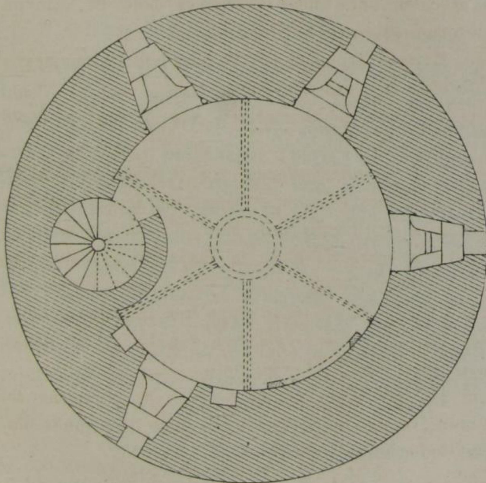
Grundriss.
